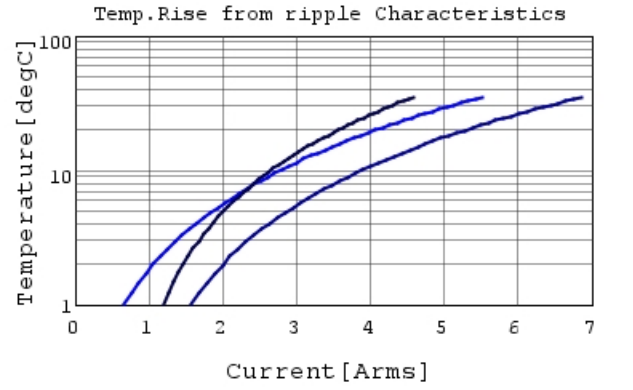
GRM32ER71C226MEA8 Temp.rise 80kHz
