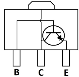
SOT-89
