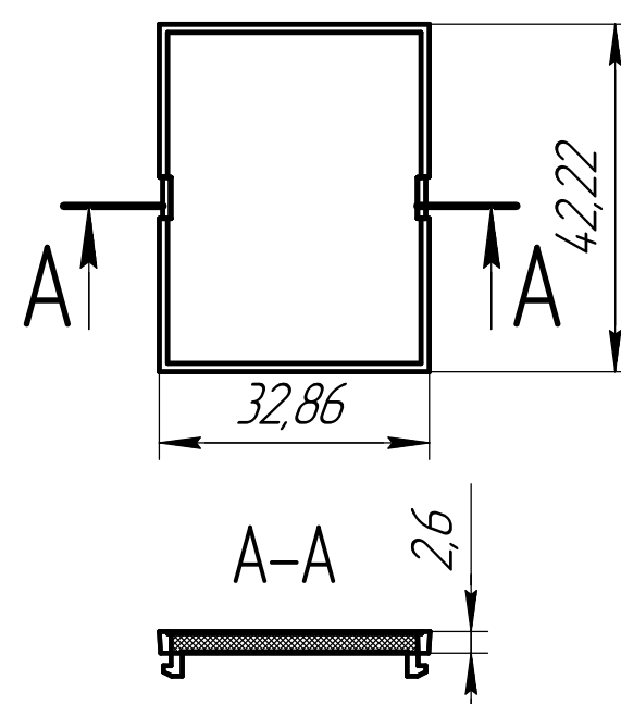
Крышка
