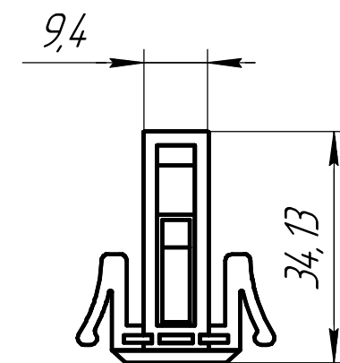
Крепление на рейку
