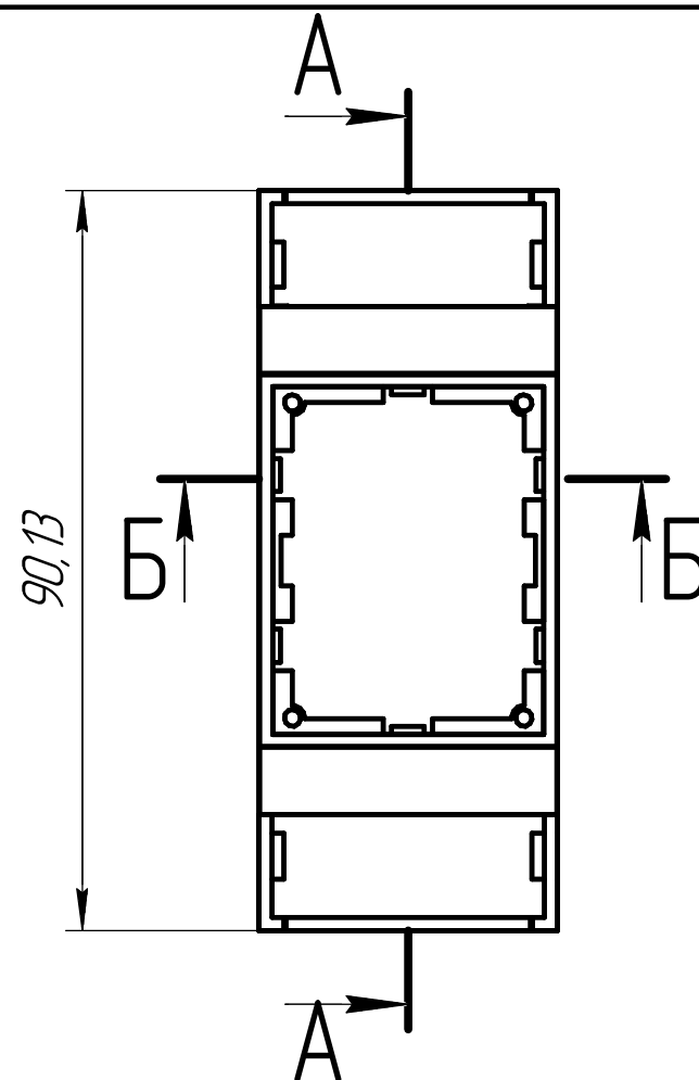
Корпус
