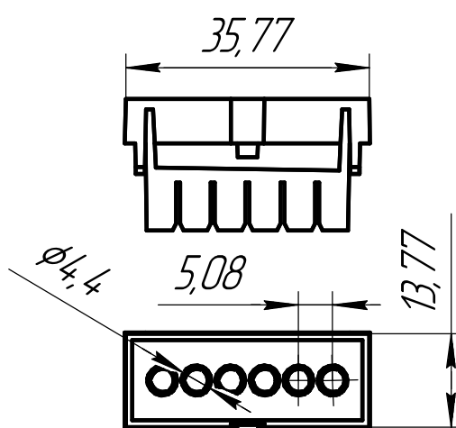
Заглицька 6 отверстий
