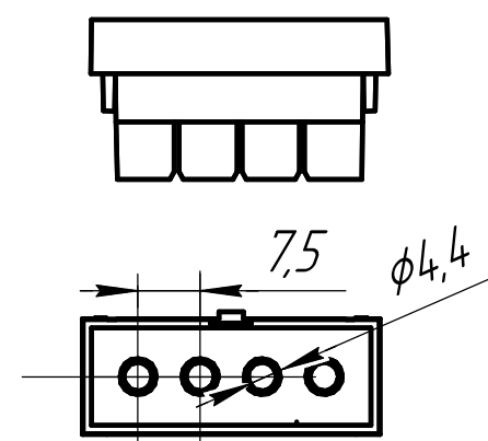
Заглушка 4 отверстия (опционально)
