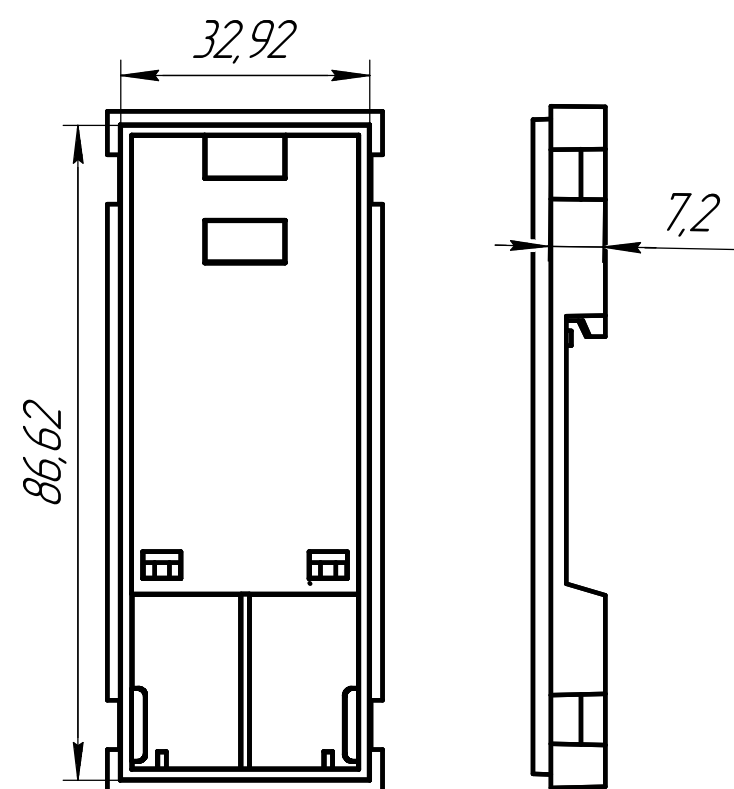
Основание
