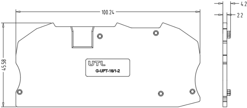
外形尺寸公差
