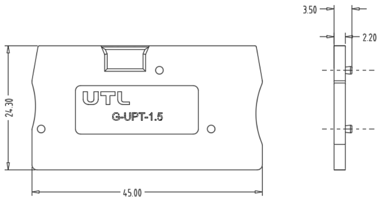
外形尺寸公差
