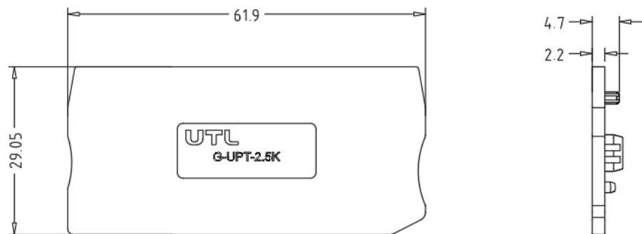
外形尺寸公差
