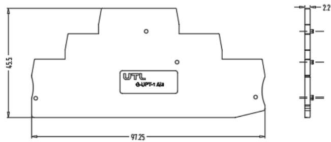
外形尺寸公差
