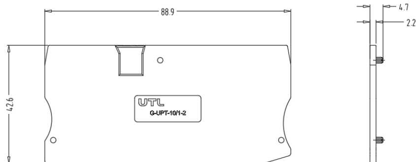
外形尺寸公差
