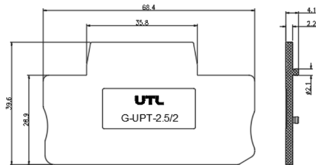
外形尺寸公差
